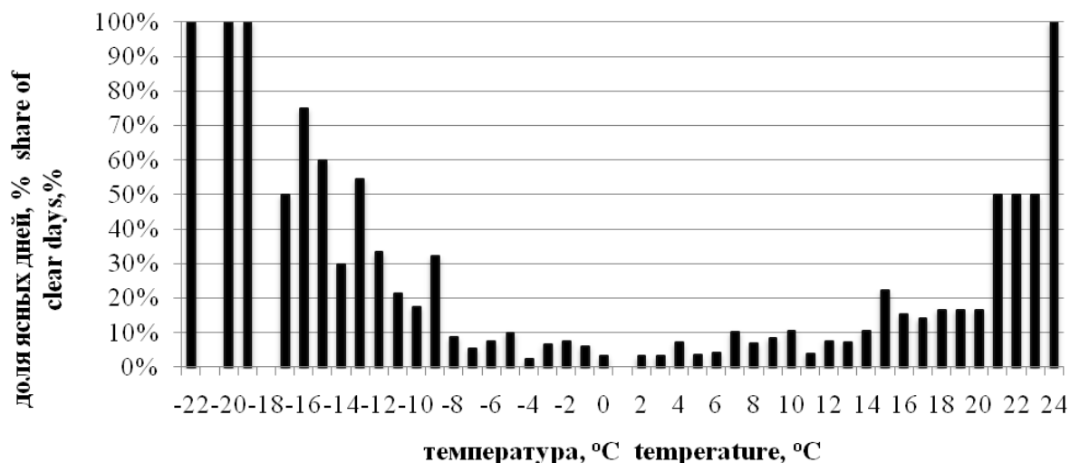
Рисунок 4. Зависимость количества ясных дней от температуры воздуха в Москве за период октябрь-январь Figure 4. The dependence of the number of clear days on air temperature in Moscow for the period October-January
