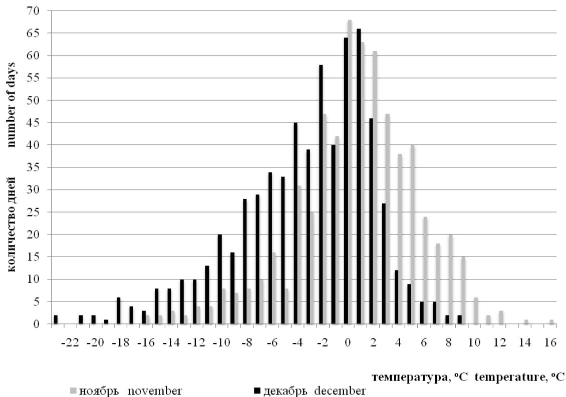
Рисунок 3. Температура воздуха в Москве в ноябре и декабре за период с 1997 по 2017 гг. Figure 3. Air temperature in Moscow in November and December for the period from 1997 to 2017
