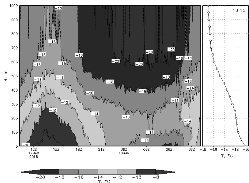
Рисунок 5. Вертикальное распределение температуры в Москве [15]. Время 10-10. Координаты профилера: ФГБУ Центральная аэрологическая обсерватория, Московская обл., г. Долгопрудный, ул. Первомайская, 3 ( 55^{\circ}55'32''N , 37^{\circ}31'23''E )
