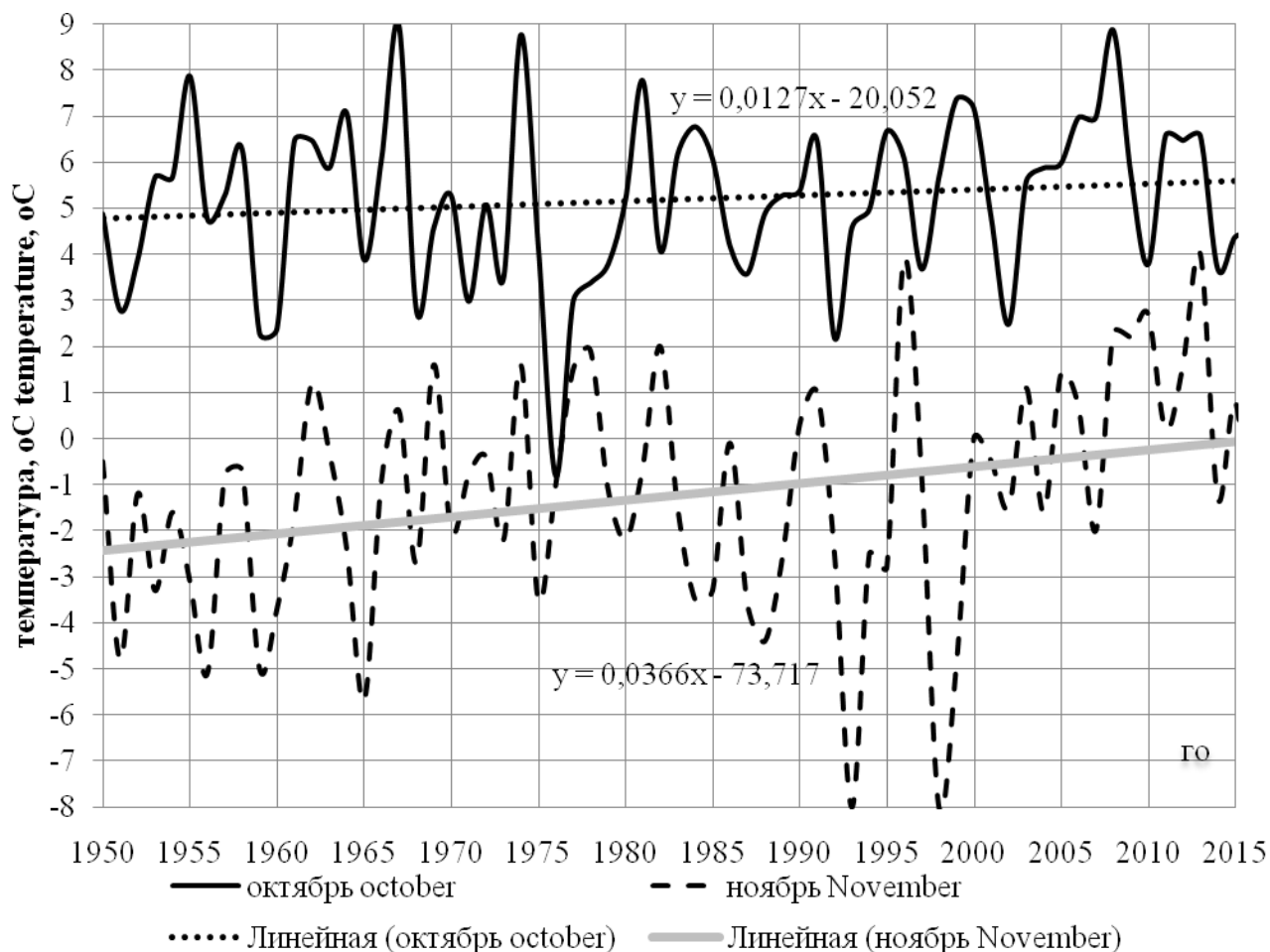
Рисунок 1. Среднемесячная температура в Москве месяцы октябрь, ноябрь за период наблюдения [11]
